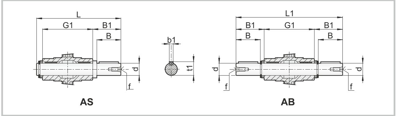
Şekil 11: Çıkış Mili
