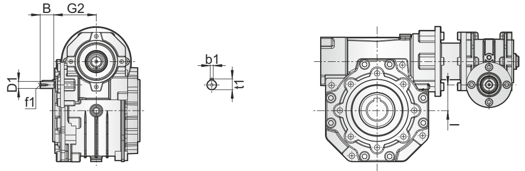
Şekil 14 - b: Giriş Mili
