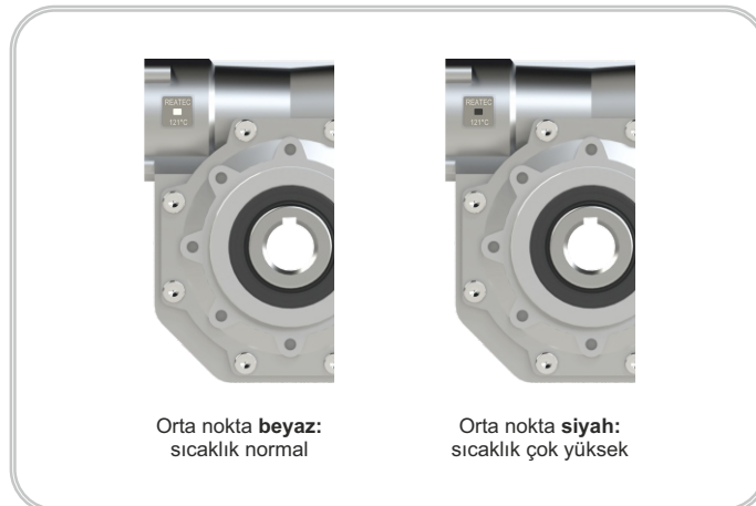
Şekil 8: Sıcaklık Etiketi
