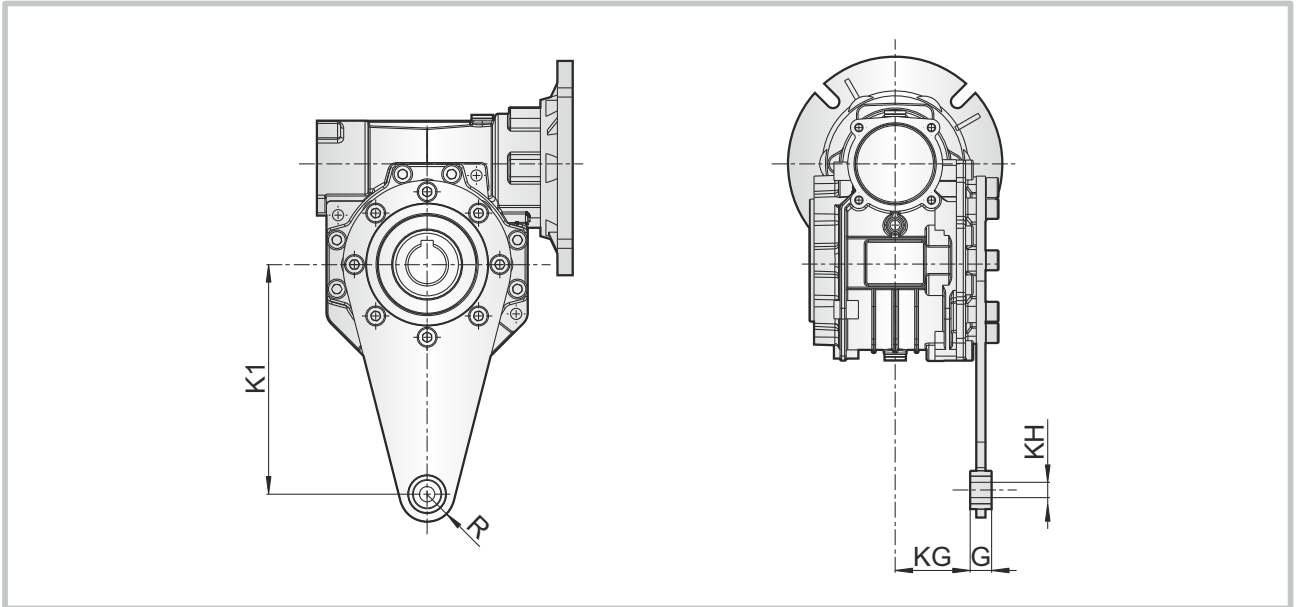
Şekil 13: Tork Kolu
