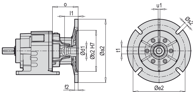
AF 202 G PAM B5/B14
